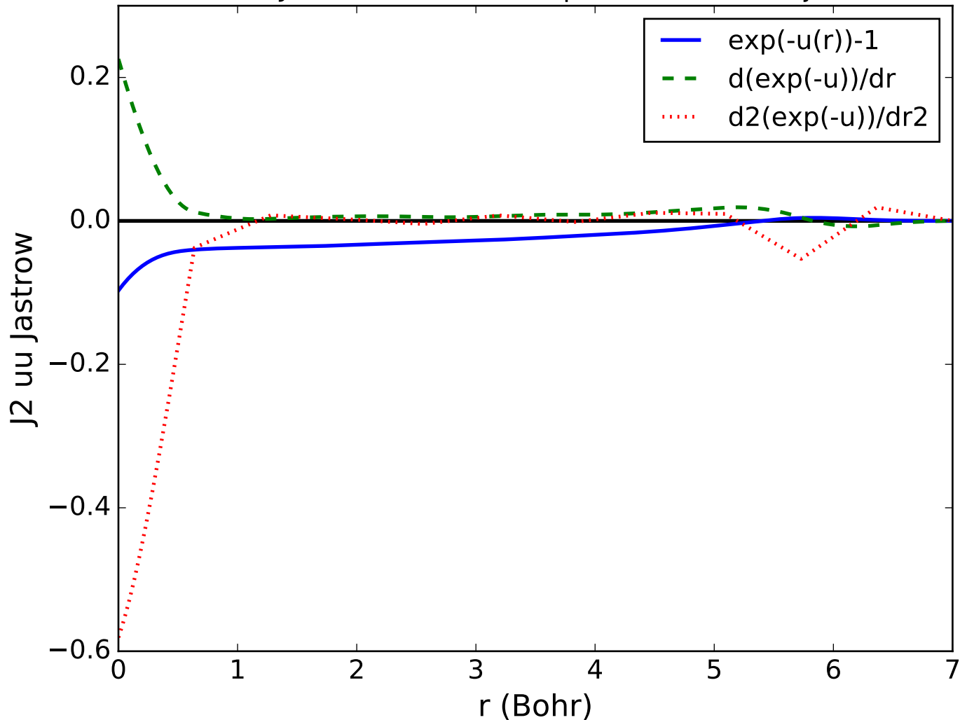
CIPSI-Jastrow/H2O/H2O-cc-pcvTz-multidet.wfj.xml
