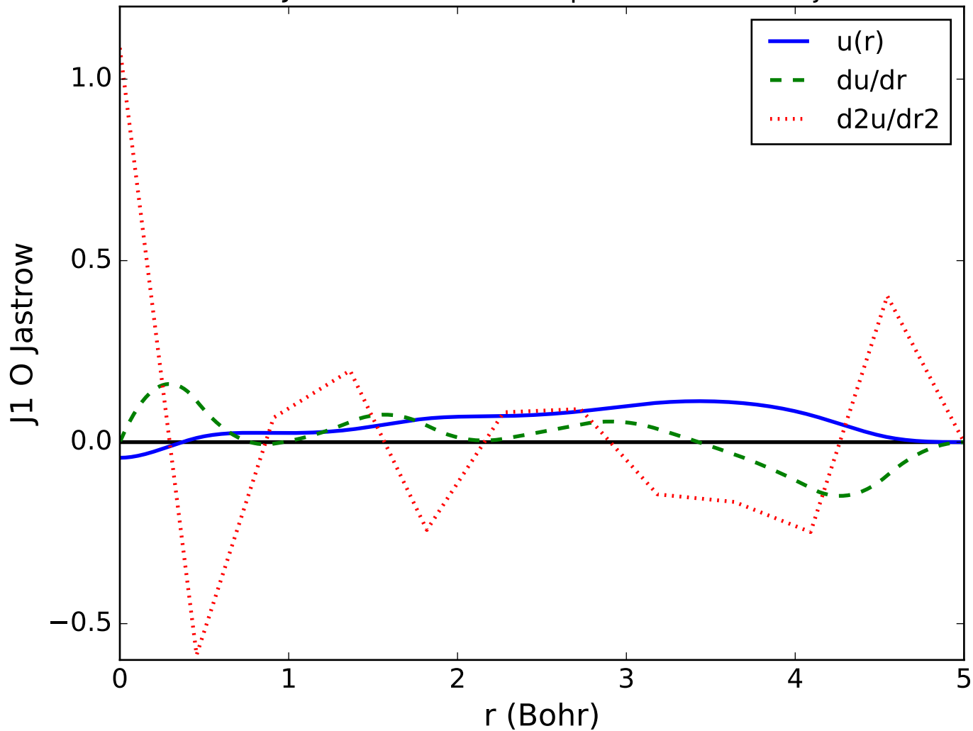
CIPSI-Jastrow/H2O/H2O-cc-pcvTz-multidet.wfj.xml
