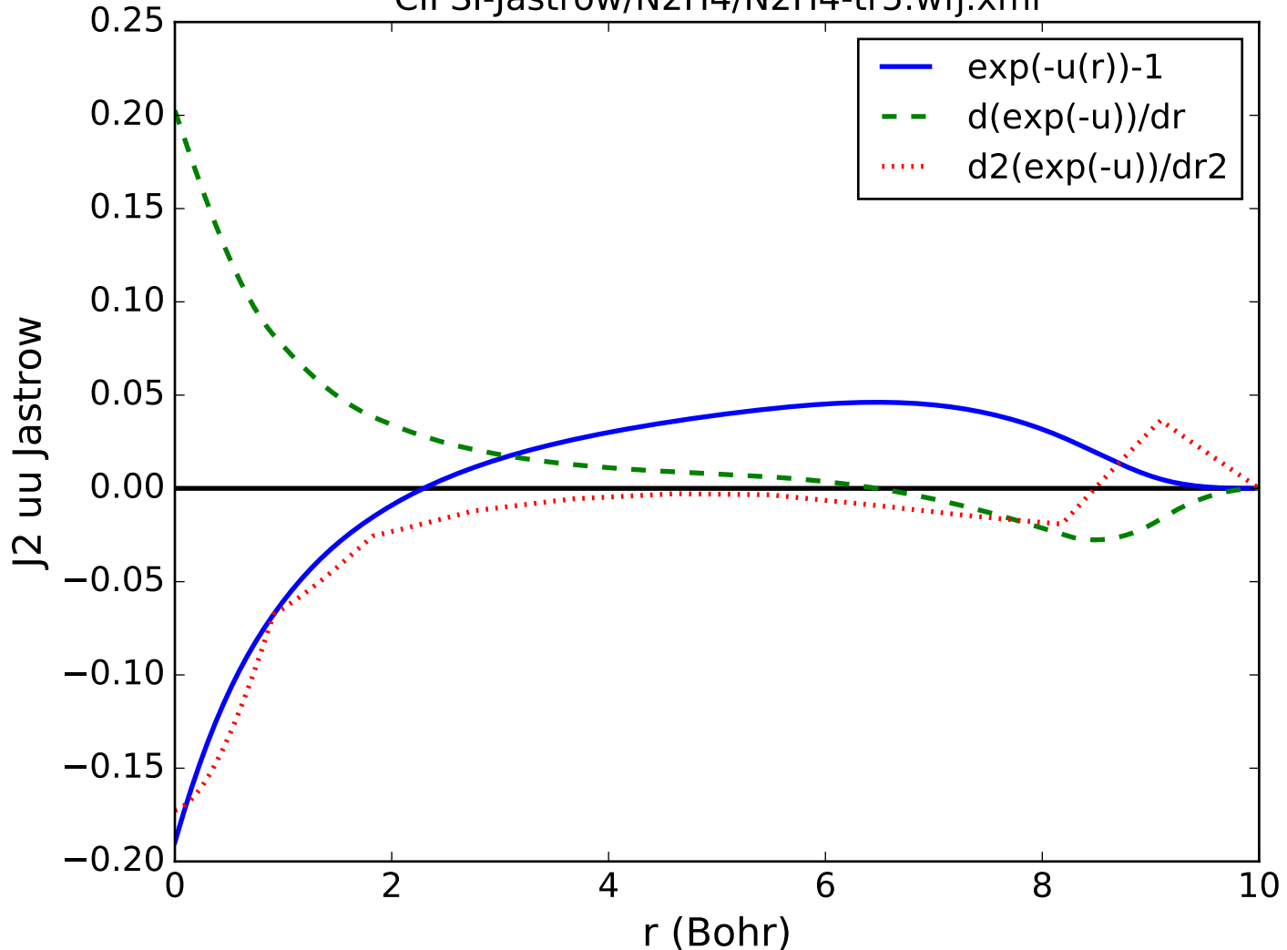
CIPSI-Jastrow/N2H4/N2H4-tr5.wfj.xml
