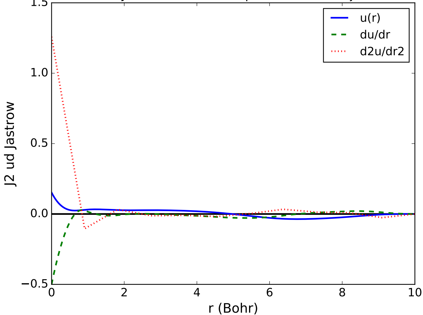
CIPSI-Jastrow/H2O/H2O-cc-pcvTz-multidet.wfj.xml
