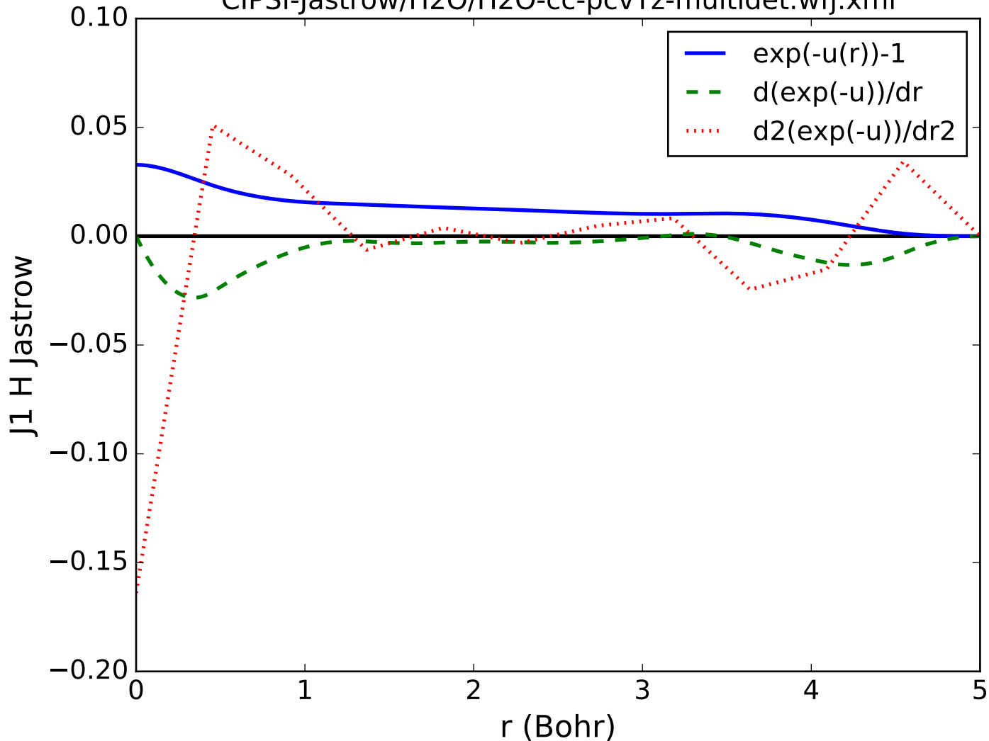
CIPSI-Jastrow/H2O/H2O-cc-pcvTz-multidet.wfj.xml
