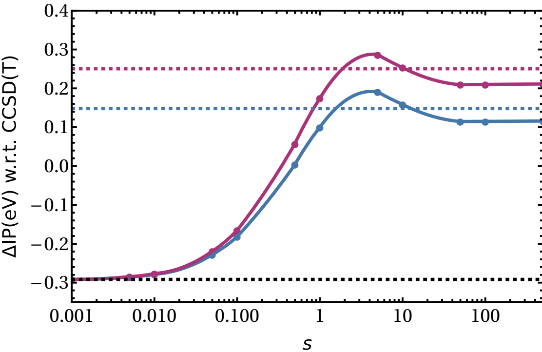
Li 2
