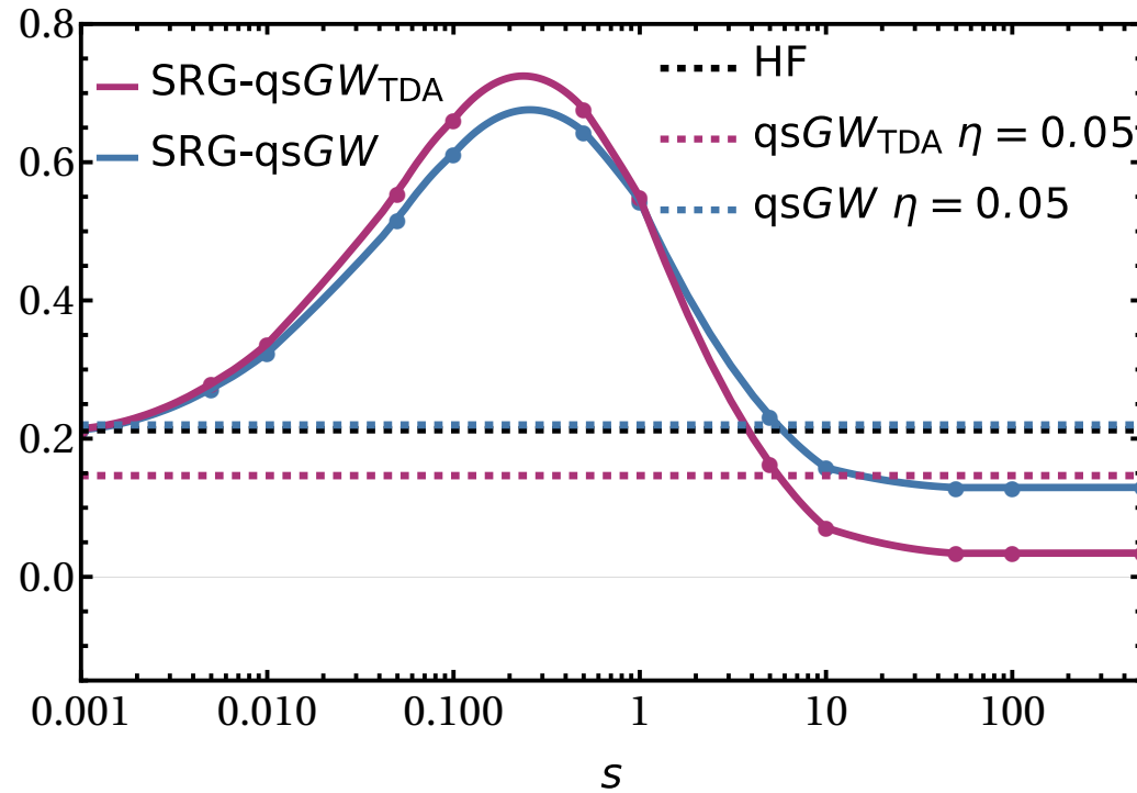
LiH
