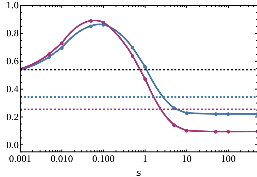
BeO
