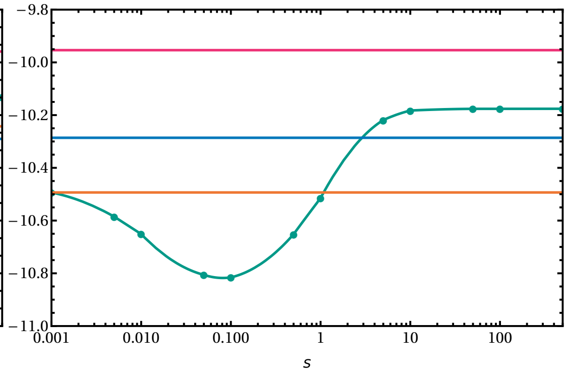
BeO
