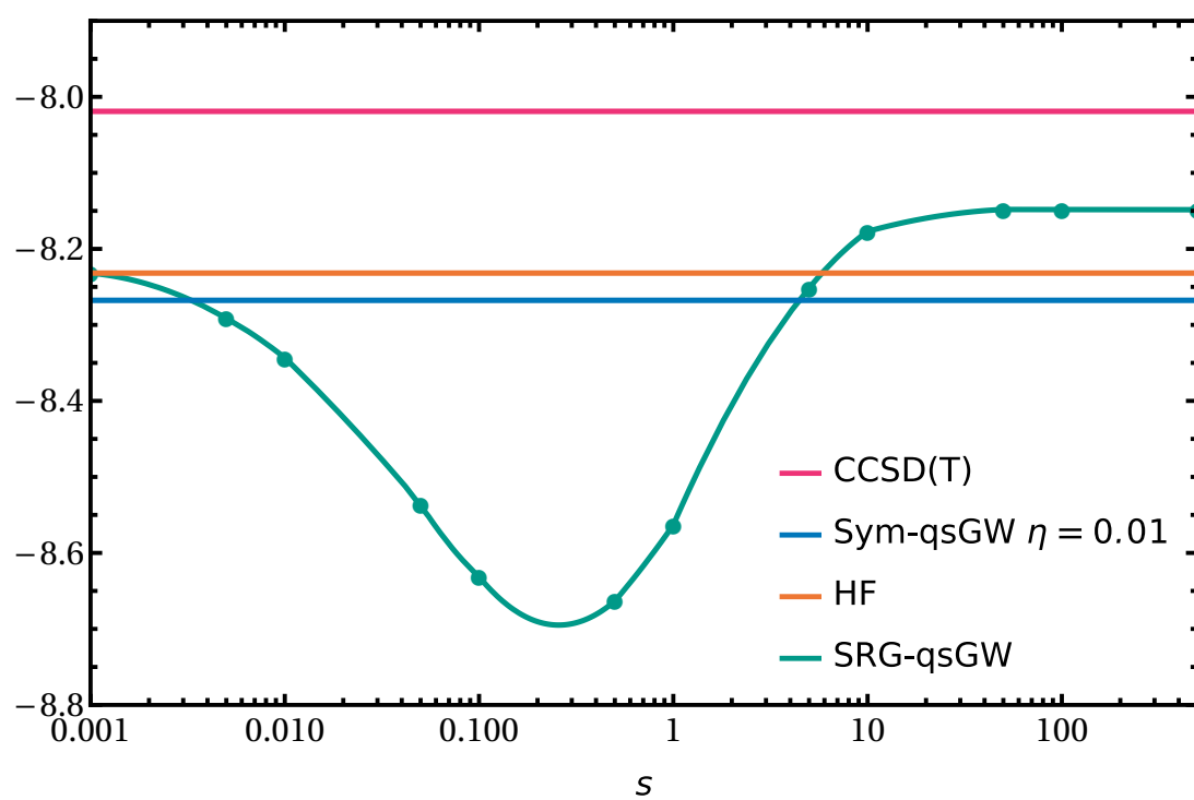
LiH
