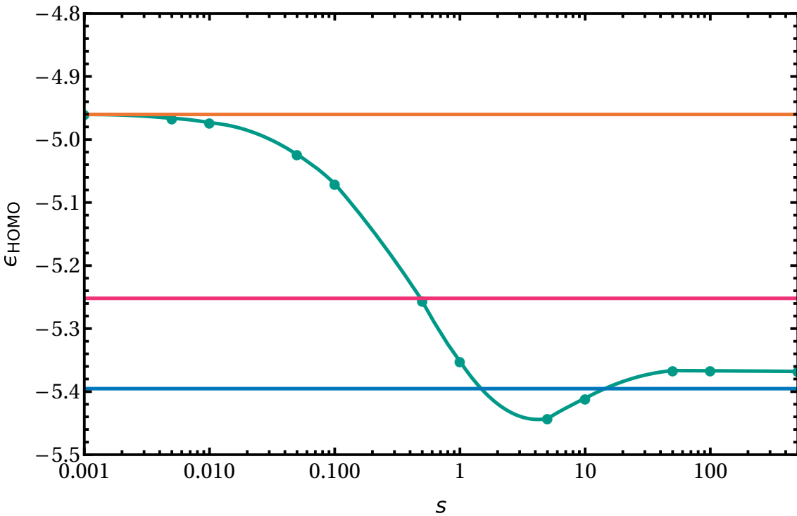
Li 2
