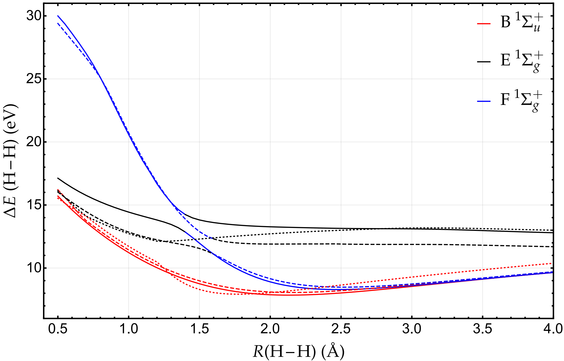
(SF-)BSE@G 0 W 0 vs EOM-CCSD
