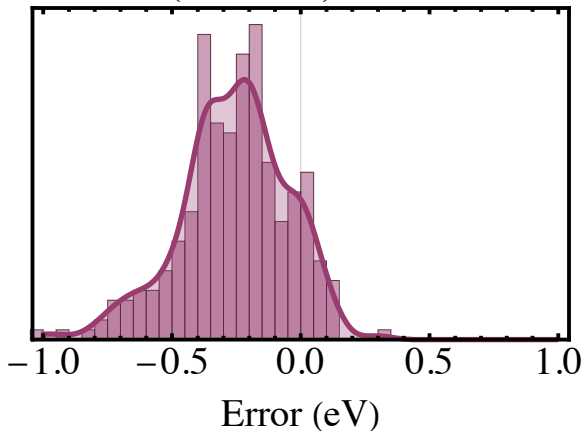
CASPT2(NOIPEA) MAE: 0.27 eV
