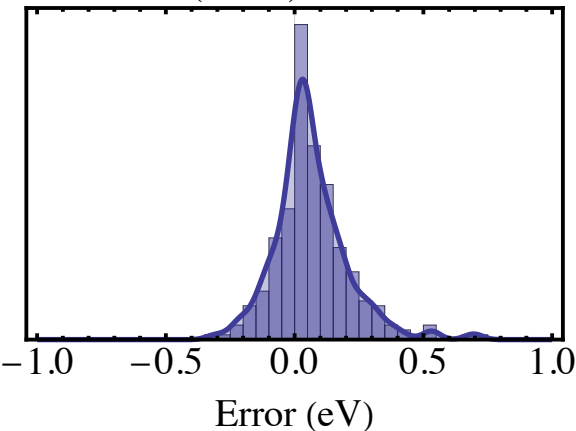
CASPT2(IPEA) MAE: 0.11 eV
