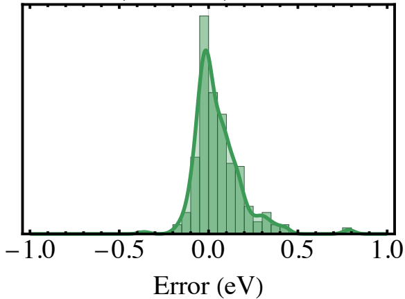
CASPT3(NOIPEA) MAE: 0.09 eV
