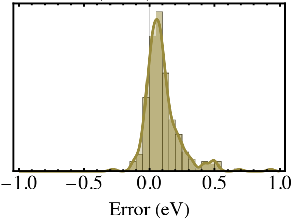
CASPT3(IPEA) MAE: 0.11 eV
