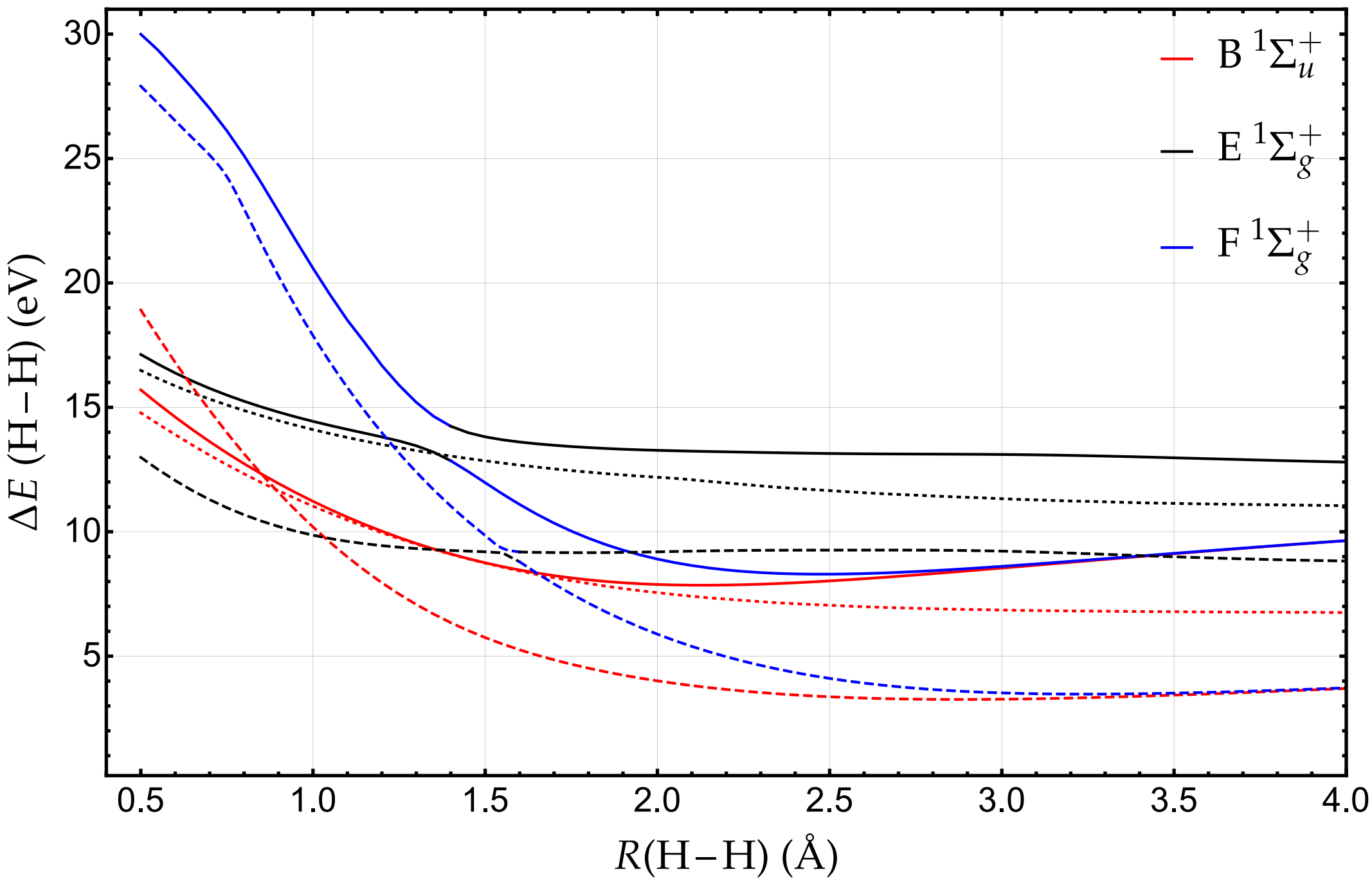
(SF-)TD- \omega B97X-D vs EOM-CCSD
