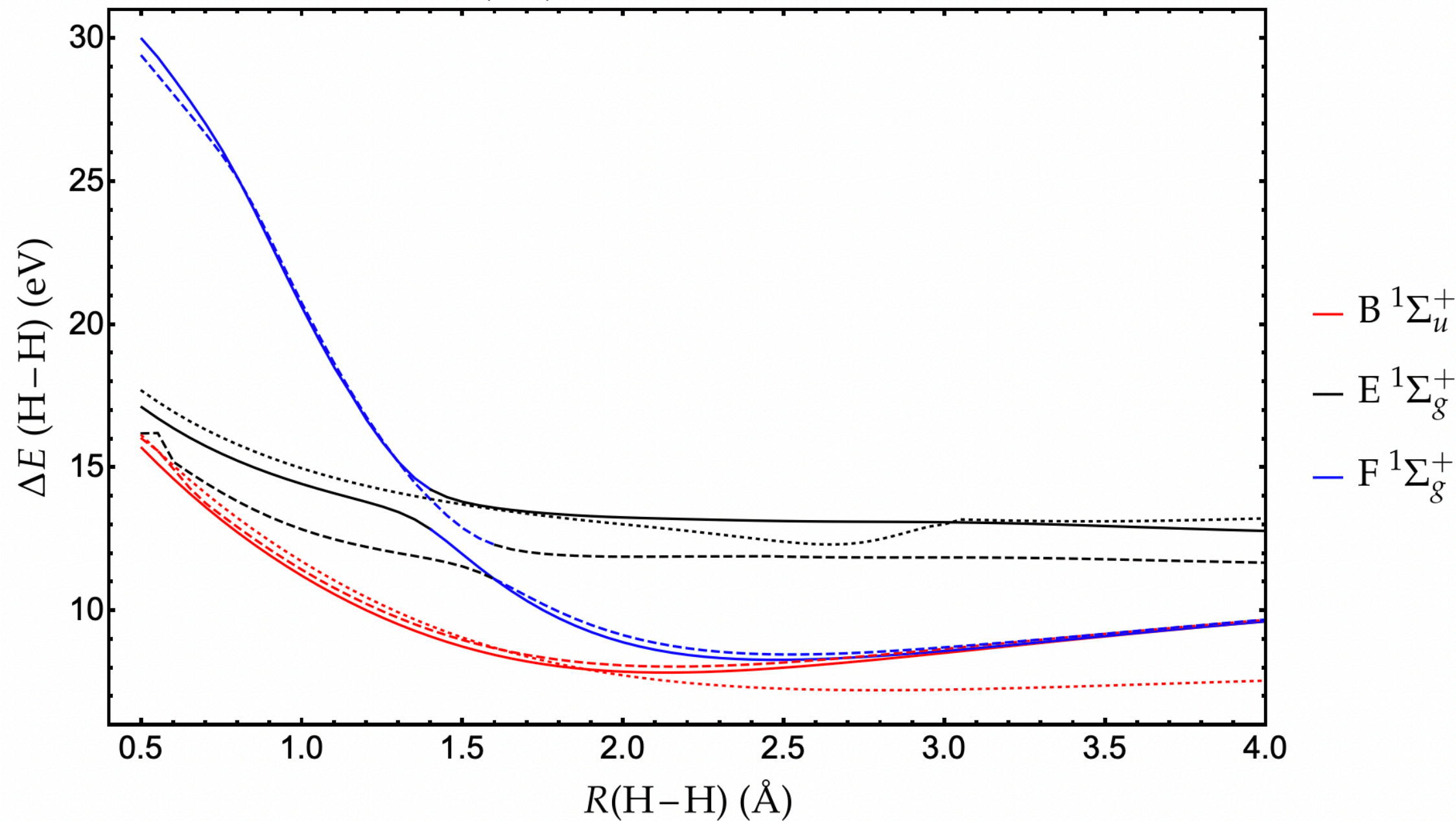
(SF-) BSE vs EOM-CCSD
