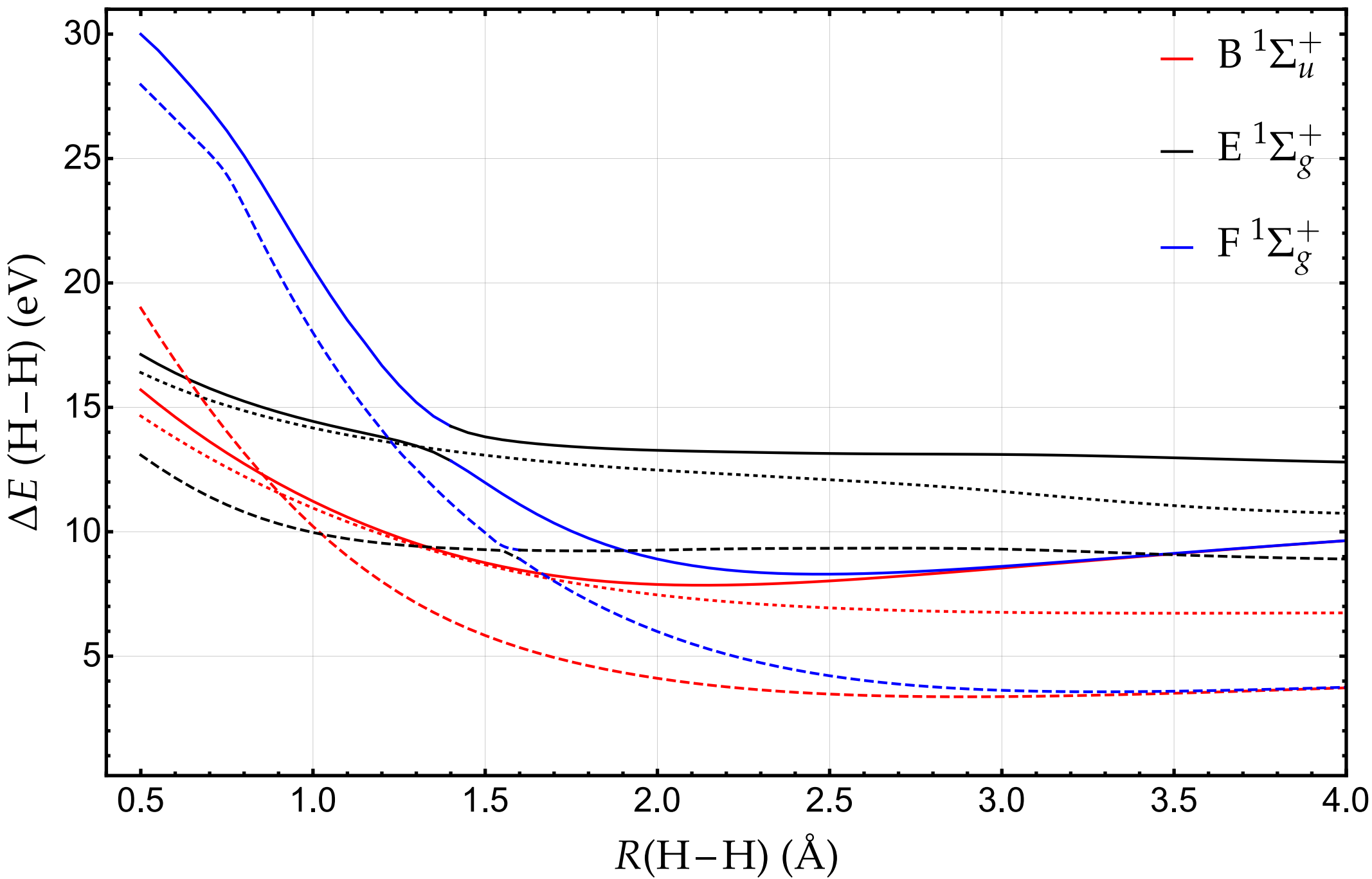
(SF-)TD-CAM-B3LYP vs EOM-CCSD
