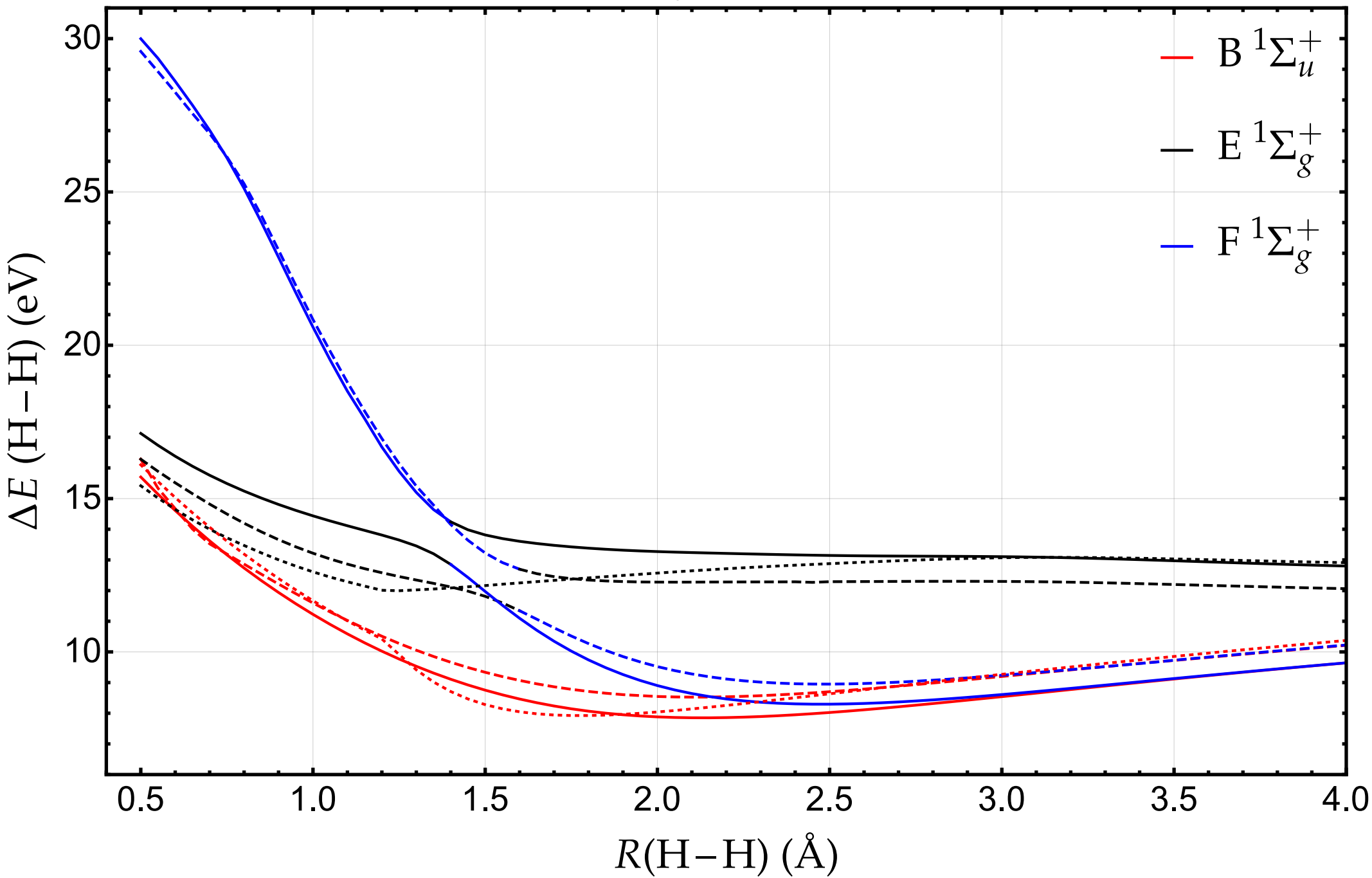
(SF-)dBSE@G 0 W 0 vs EOM-CCSD
