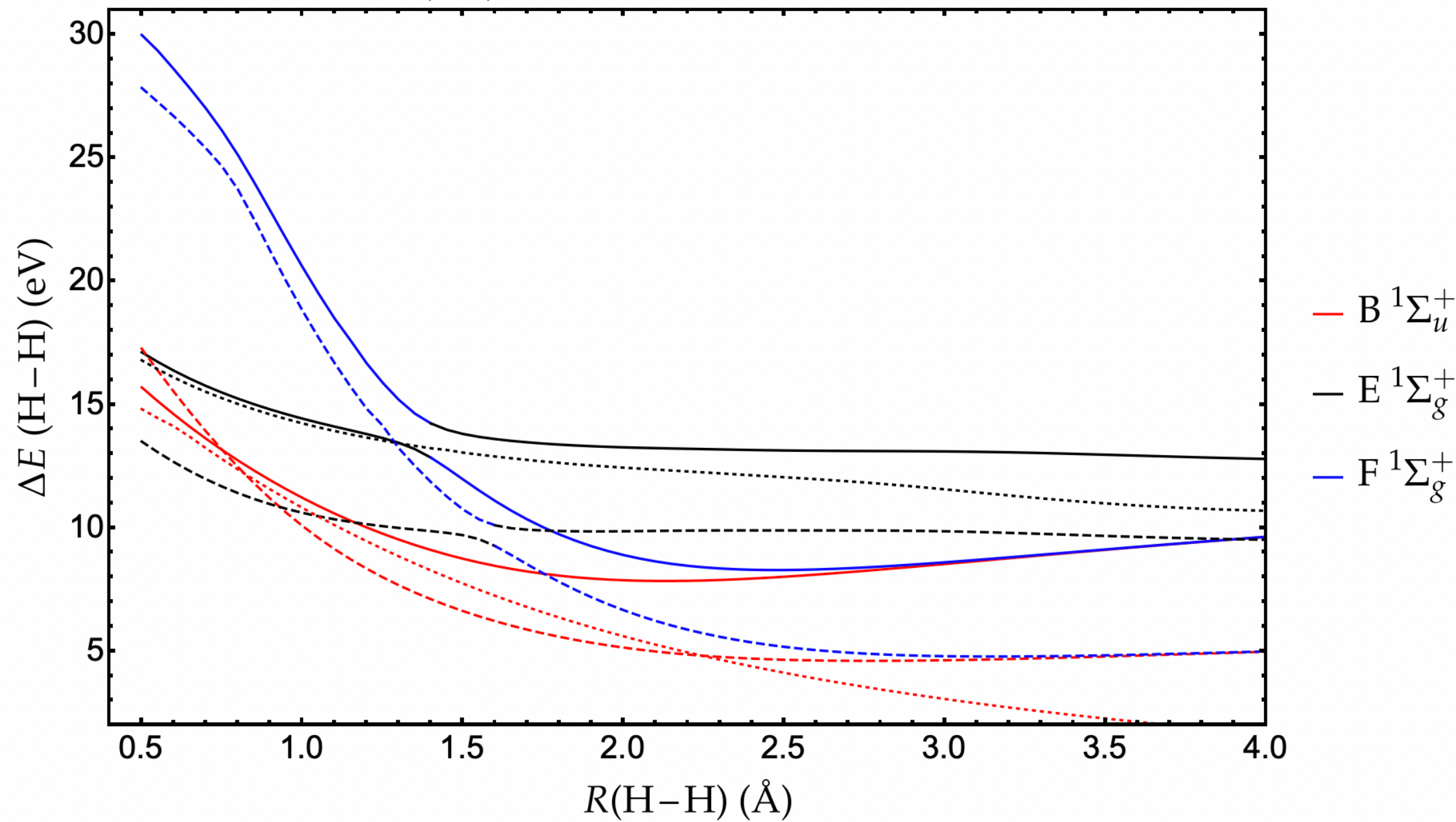
(SF-) BH&HLYP vs EOM-CCSD
